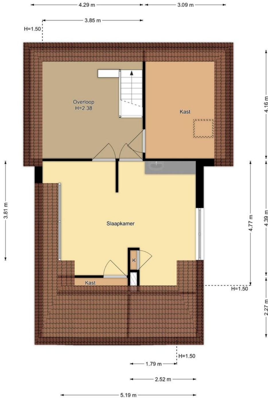
2e Verdieping Vinkenbaan 58, Bloemendaal R.M. Vastgoedpresentatie| Aan deze plattegrond kunnen geen rechten worden ontleend
